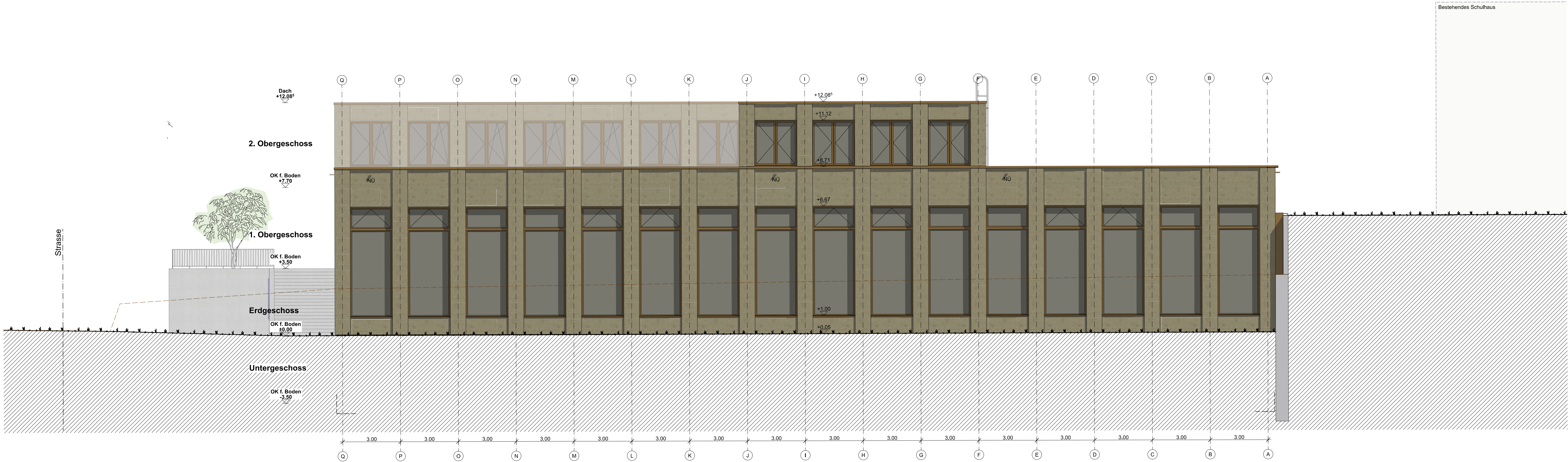
Ansicht Südwest
